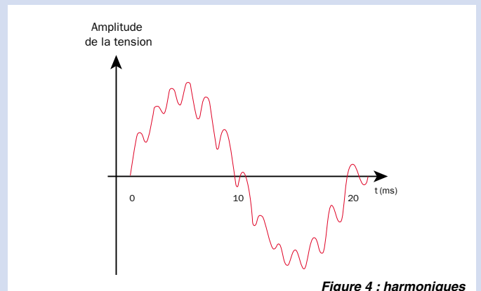
Figure 4 : harmoniques
